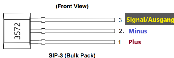
Abbildung 3: Hallsensor AH3572
