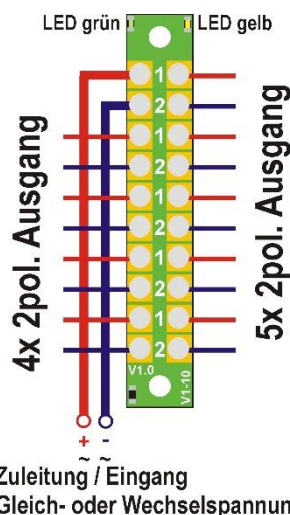
Abbildung 1: V1-10-LED
